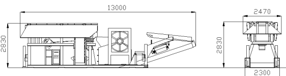
GRM-FP 750 DIMENSIONI IN CONFIGURAZIONE DI LAVORO E DI TRASPORTO
