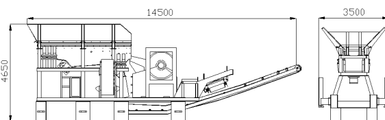
GRM-FP 750 DIMENSIONI IN CONFIGURAZIONE DI LAVORO E DI TRASPORTO
